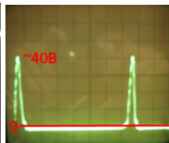
C-Z, 20V/50us клетка B-Z, 20V/50us клетка A-Z, 5V/50us клетка Out HV – импульс 15..20us 6..8KV (при R2=5.1Ом) Потребление от 6V примерно 600мА (3.6W). Далее уточнение выхода с R2=5.1Ом и нагрузкой (щуп) на 6.9МОм:
