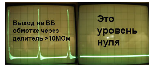
C-Z, 20V/50us клетка B-Z, 20V/50us клетка A-Z, 5V/50us клетка Out HV – импульс 15..20us 6..8KV (при R2=5.1Ом) Потребление от 6V примерно 600мА (3.6W). Далее уточнение выхода с R2=5.1Ом и нагрузкой (щуп) на 6.9МОм:
